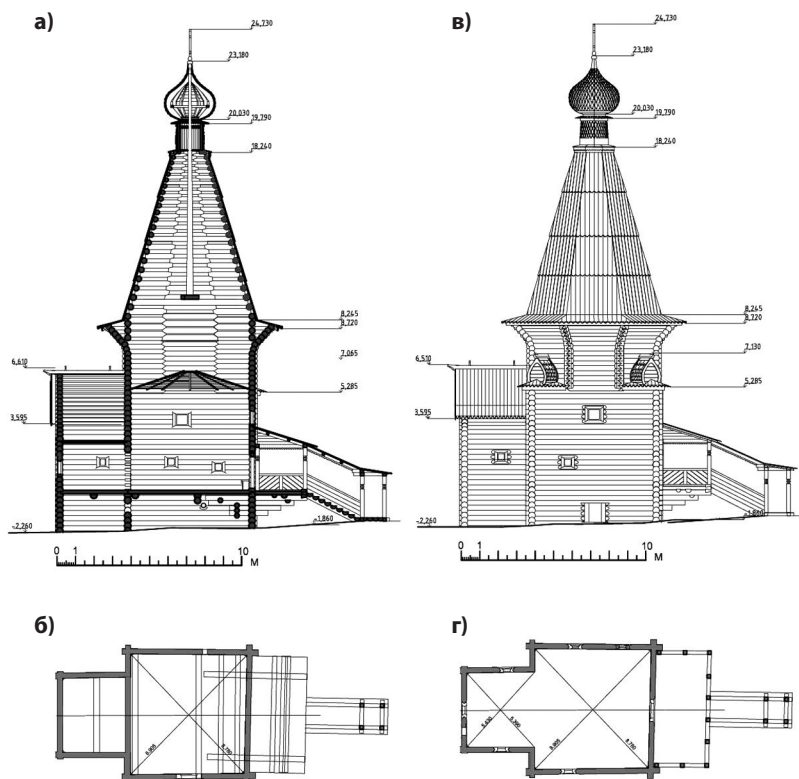
Никольская церковь. 1-й строительный этап (1648). Продольный разрез (а), план на уровне подклета (б), северный фасад (в), план (г). Обмеры Д. Ш. Якуповой, 2012 г.
