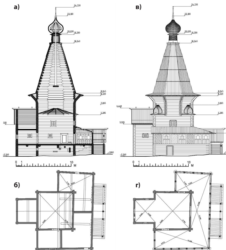
Никольская церковь. 2-й строительный этап (1760-е гг.) Продольный разрез (а), план на уровне подклета (б), северный фасад (в), план (г). Обмеры Д. Ш. Якуповой, 2012 г.
