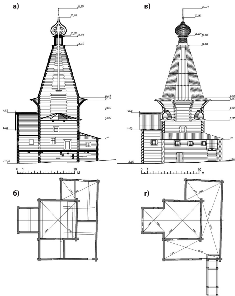
Никольская церковь. 3-й строительный этап (сер. XIX в.). Продольный разрез (а), план на уровне подклета (б), северный фасад (в), план (г). Обмеры Д. Ш. Якуповой, 2012 г.
