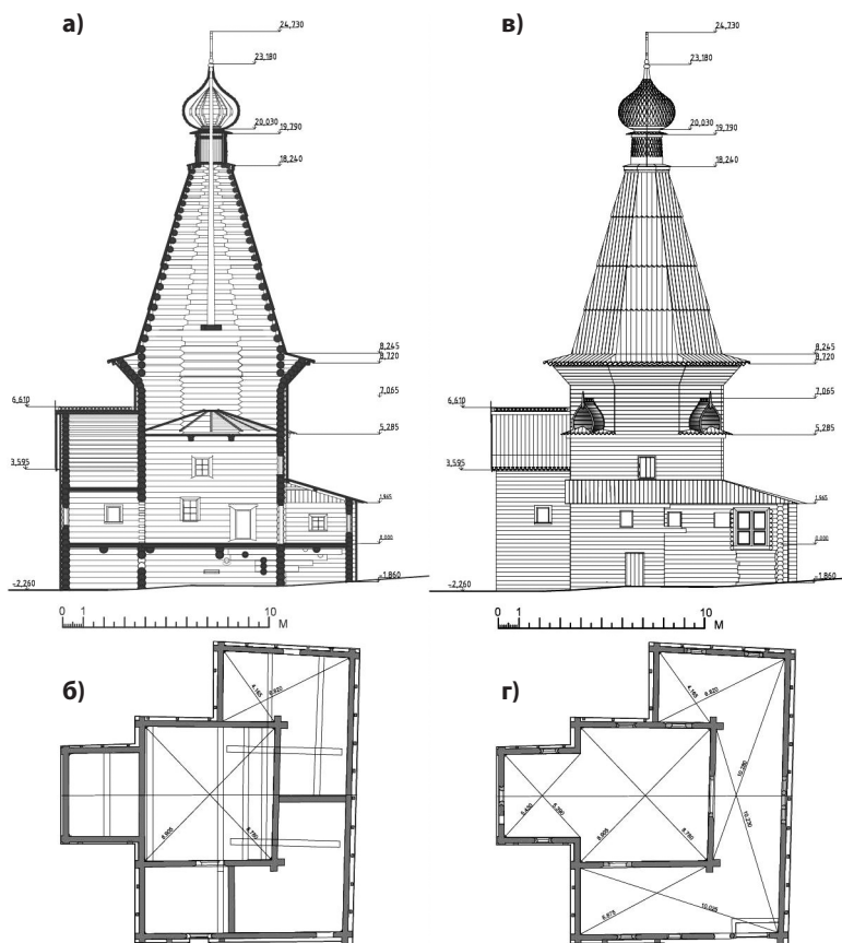
Никольская церковь. 4-й строительный этап (1875). Продольный разрез (а), план на уровне подклета (б), северный фасад (в), план (г). Обмеры Д. Ш. Якуповой, 2012 г.
